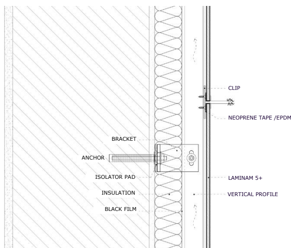
Вертикальный разрез
